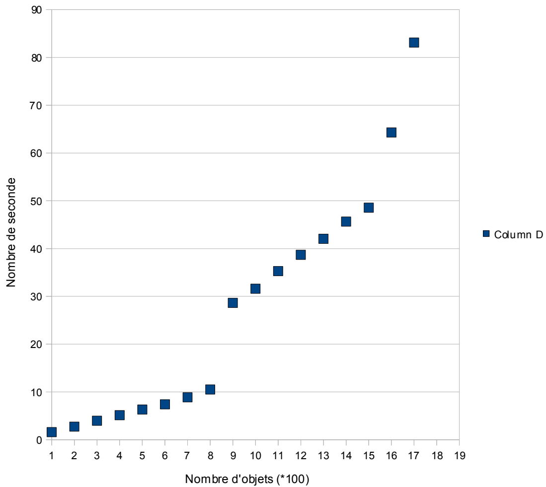
Temps requête pour 10 000 éléments (sans index spatial)
